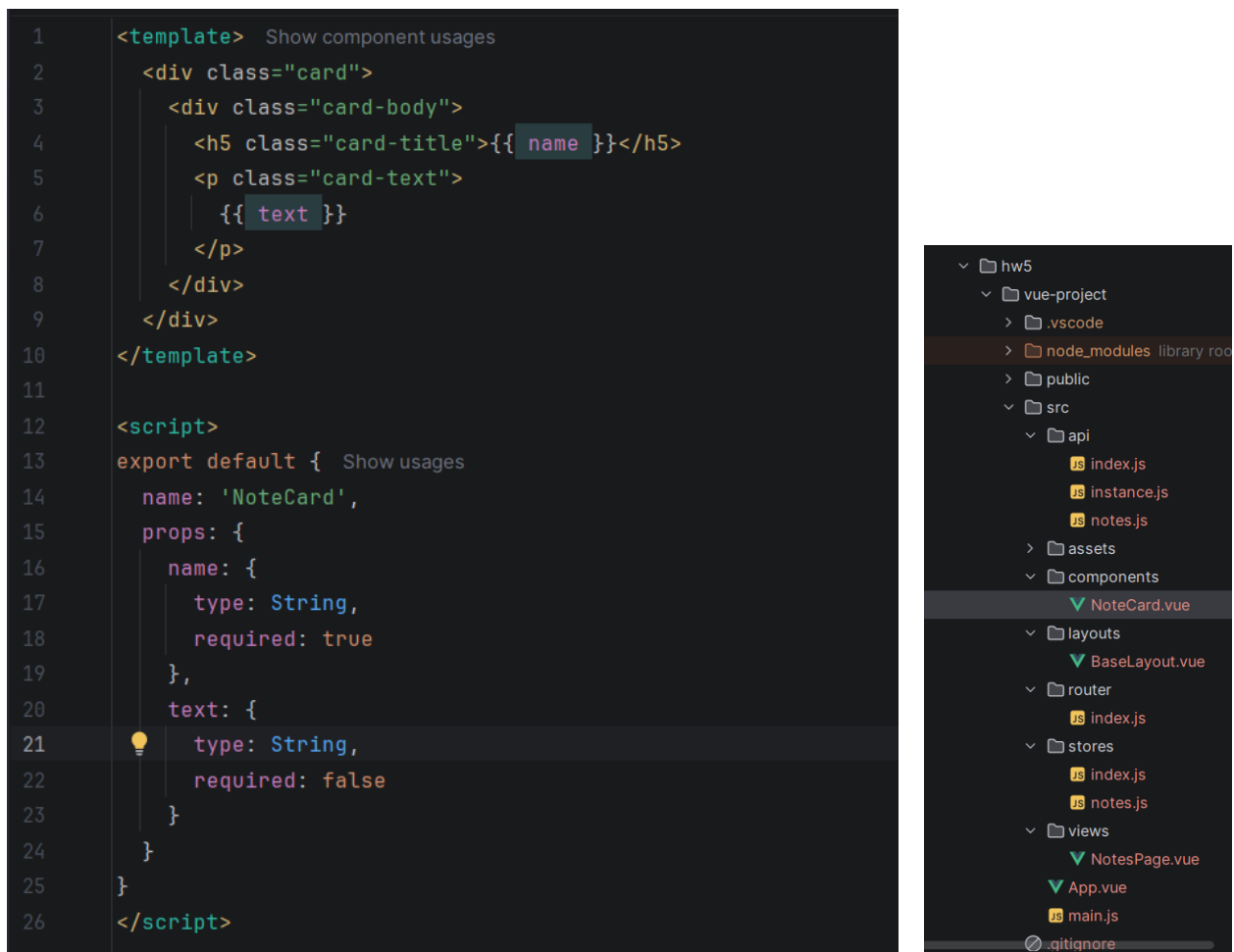
Фигура 3. Код src/components/NoteCard.vue
